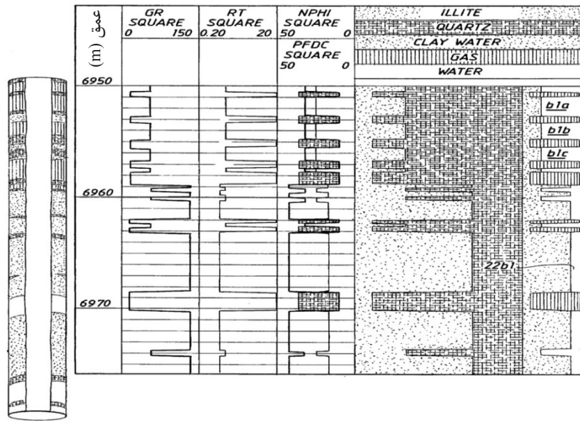
شکل ۴ نمایی از نتایج آنالیز با روش نمودارهای تصویرگر در توالی ماسه شیل نازک لایه [۵].
