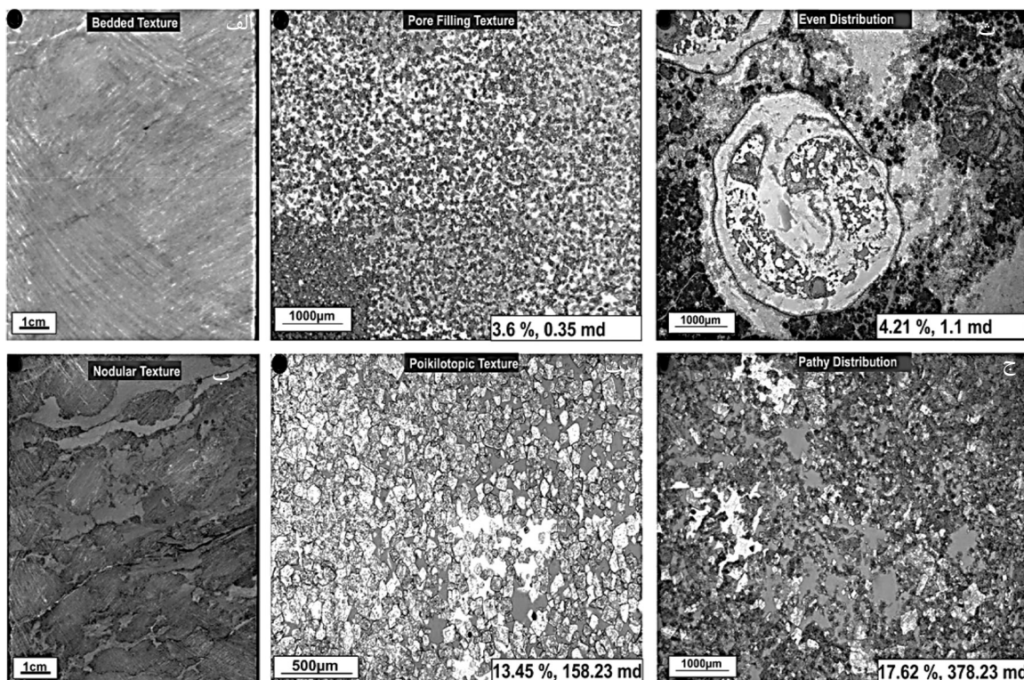
شکل ۲ تصاویر مغزه (الف و ب) و مقاطع نازک میکروسکوپی (پ، ت، ث و ج) بافت و توزیع انیدریت در توالی دولومیتی-انیدریتی سازند عرب، (الف) بافت لایه‌ای، (ب) نودولار، (پ) پرکننده تخلخل، (ت) پوکیلوتوپیک، (ث) توزیع یکنواخت، (ج) توزیع پراکنده. تصاویر پ در PPL و ت، ث و ج در XPL
