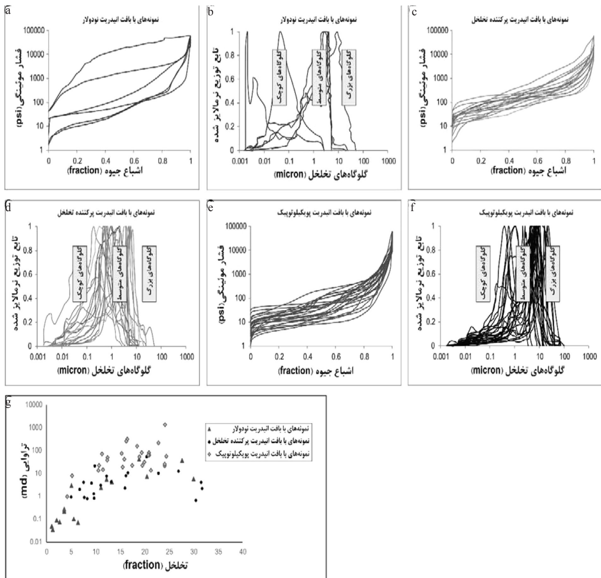
شکل ۴ منحنی‌های فشار موئینه (a-c-e)، توزیع گلوله‌های تخلخل (b-d-f) و نیز توزیع تخلخل-تراوایی (g) براساس گروه‌بندی نمونه‌ها بر مبنای بافت انیدریت. (a-b) نمونه‌های با بافت انیدریت نودولار، (c-d) نمونه‌های با بافت انیدریت پرکننده تخلخل، (e-f) نمونه‌های با بافت انیدریت پویکیلو توپیک، (g) توزیع تخلخل-تراوایی در نمونه‌هایی با بافت متفاوت انیدریت.
