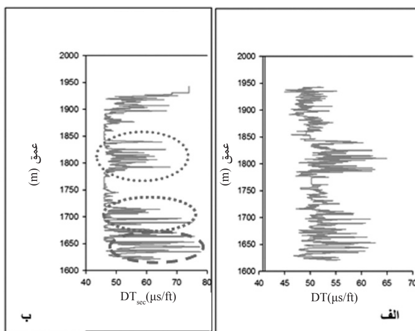
شکل ۶- مقایسه نمودار صوتی: مشتق گرفتن در سطح اول (شکل الف) و مشتق گرفتن در سطح دوم (شکل ب). زون‌های شکسته در حالت دوم بهتر خود را نشان می‌دهند.
