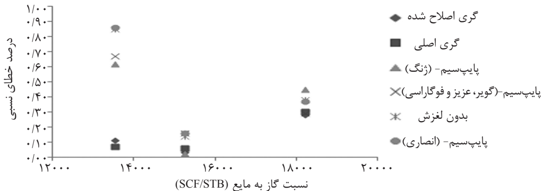
شکل ۸- درصد خطای نسبی روابط نرم افزار پایپ سیم نسبت به تغییر گاز به میعانات
