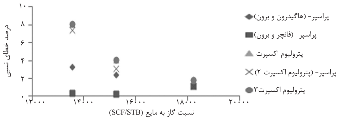
شکل ۶- درصد خطای نسبی روابط نرم افزار پراسپیر نسبت به تغییر گاز به میعانات
