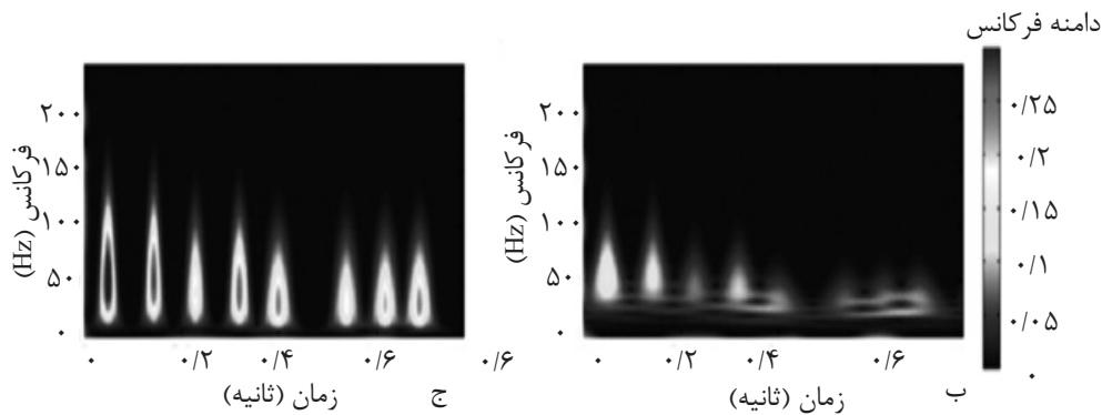
شکل ۲- سیگنال مصنوعی با صفحه زمان- فرکانس (الف) سیگنال ناپایا مصنوعی موجک ریکر با فرکانس‌های ۳۵، ۲۵ و ۴۵ Hz؛ (ب) نمودار صفحه زمان- فرکانس تبدیل S استاندارد مربوط به ج) نمودار صفحه زمان- فرکانس تبدیل S تعمیم یافته مربوط به شکل ۲ (الف).
