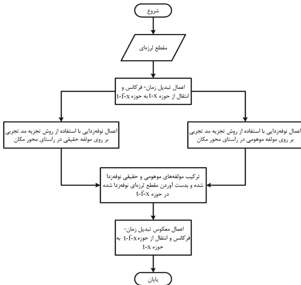
شکل ۴- نمودار گردش‌تضعیف نوفه تصادفی با استفاده از ترکیب تبدیل زمان-فرکانس و تجزیه مد تجربی
