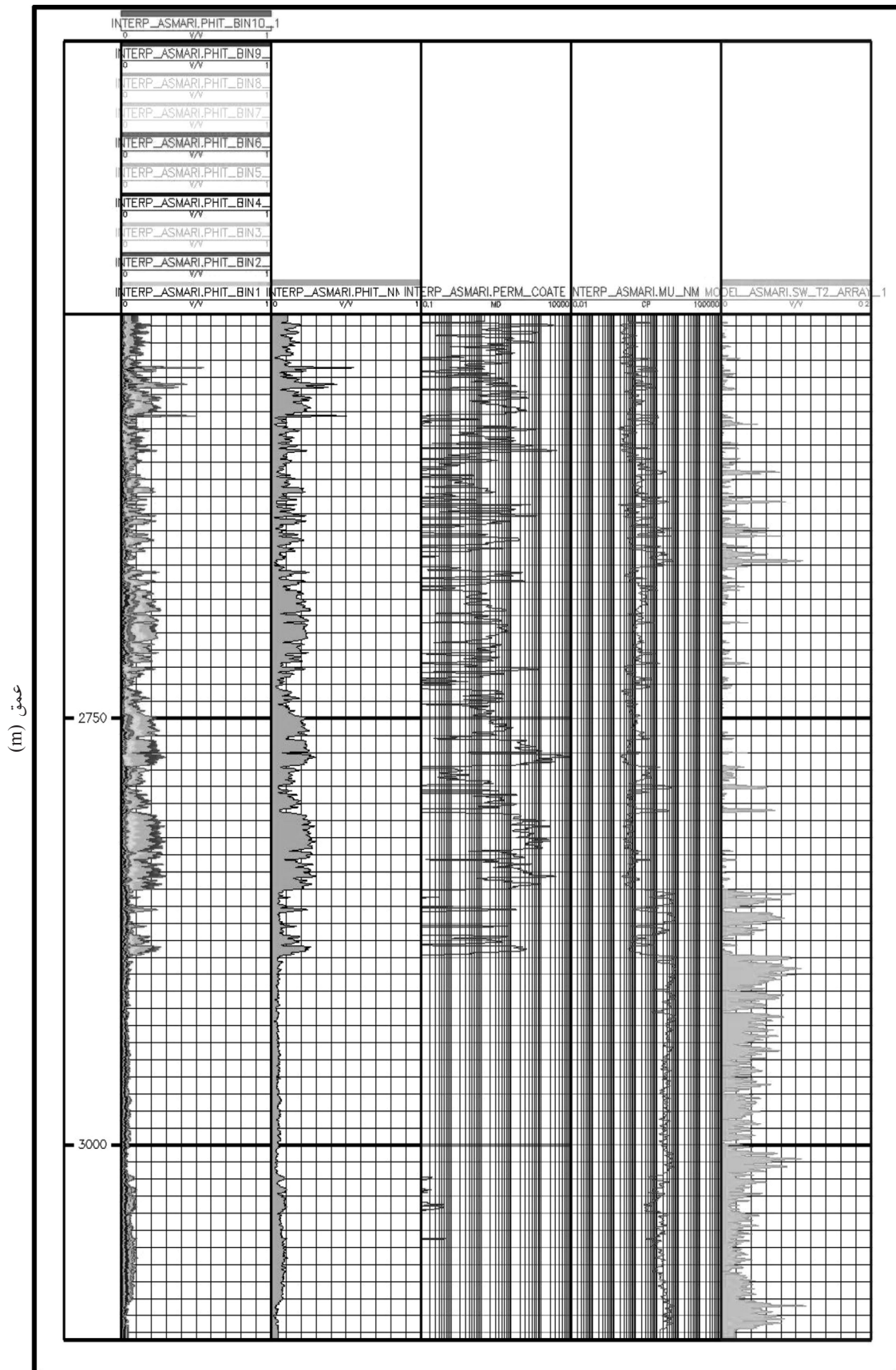
شکل ۲- پارامترهای پتروفیزیکی سازند آسماری که به ترتیب در تراک ۲ تا ۶ تخلخل بازه‌های مختلف، تخلخل کل، نفوذپذیری، ویسکوزیته و اشباع آب رسم شده است.
