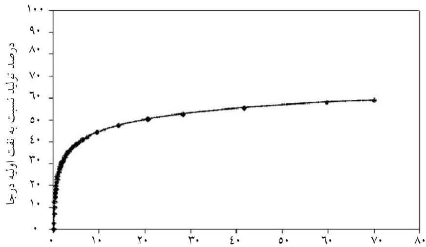
شکل ۶- تولید نفت سازند بنگستان بر حسب مقدار آب تزریقی در سنگ مخزن شماره یک
