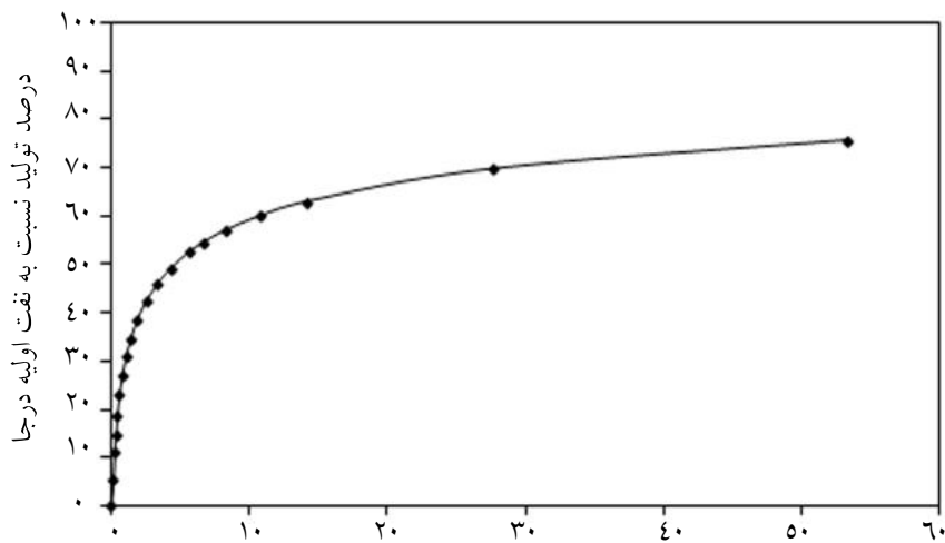
شکل ۷- تولید نفت سازند آسماری (میدان اول سازند آسماری) بر حسب مقدار آب تزریقی در سنگ مخزن شماره دو
