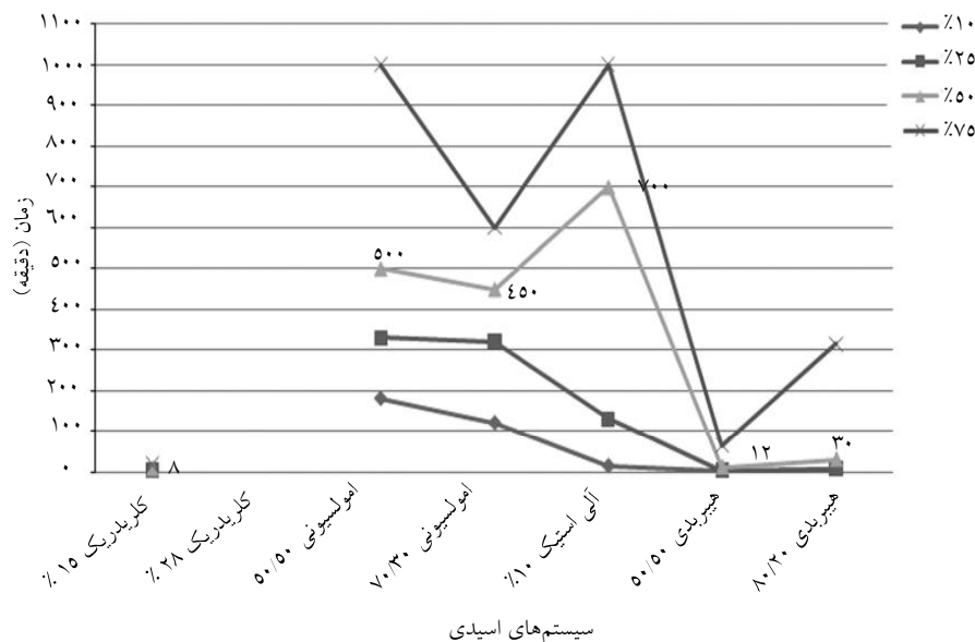
شکل ۱۹- زمان لازم برای حلالیت استاتیکی سنگ مخزن (مختلف) در دمای ۱۰۰ °C در سیستم‌های اسیدزنی مختلف
