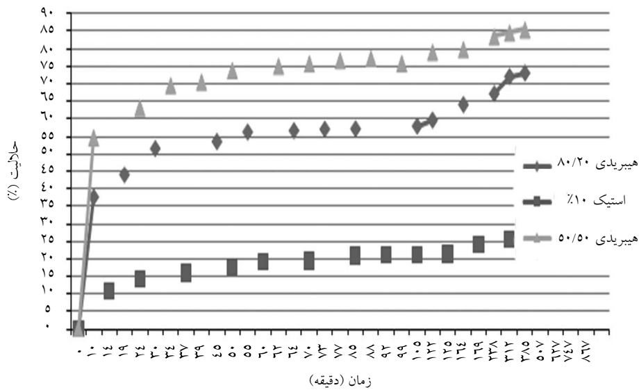
شکل ۱۰- نمودار مقایسه حالیّت استاتیکی سنگ مخزن در حضور اسیدهای هیبریدی و آلی
