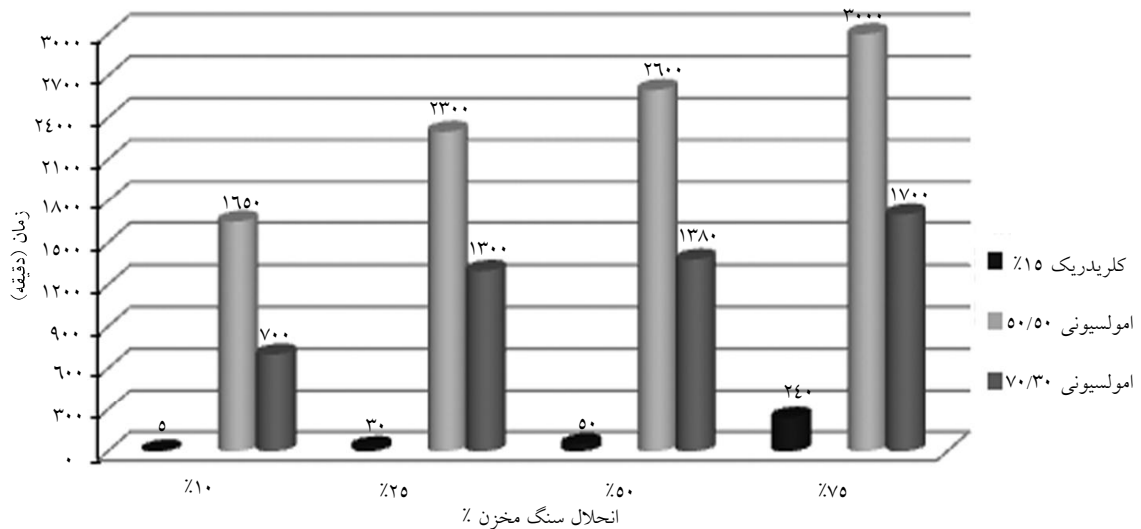
شکل ۱۳- نمودار مقایسه زمان لازم برای حلالیت استاتیکی سنگ مخزن (% مشابه) اسیدهای معدنی و امولسیونی در دمای ۶۰ °C
