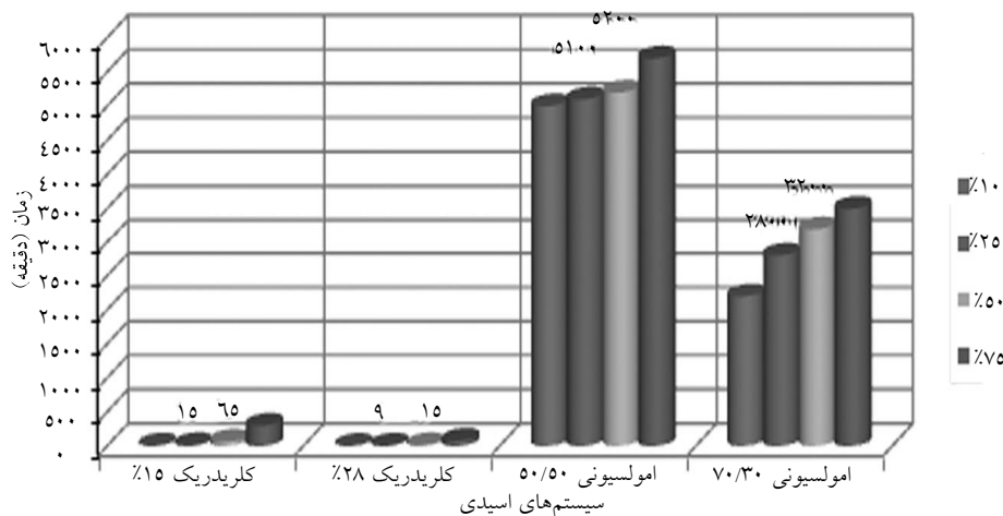
شکل ۱۲- زمان لازم برای حالیّت استاتیکی سنگ مخزن در اسیدهای مختلف در دمای ۲۵ °C
