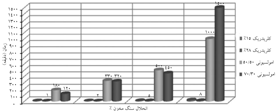
شکل ۱۴- نمودار مقایسه زمان لازم برای حلالیت استاتیکی سنگ مخزن (% مشابه) اسیدهای معدنی و امولسیونی در ۱۰۰ °C
