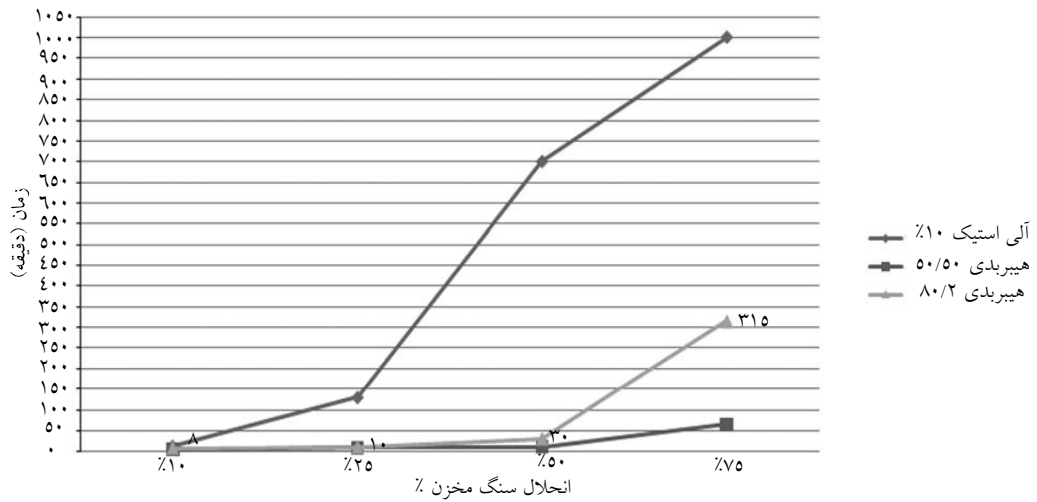
شکل ۱۵- نمودارمقایسه زمان لازم برای حلالیت استاتیکی سنگ مخزن (% مشابه) در اسیدهای آلی و هیبریدی در دمای ۱۰۰ °C
